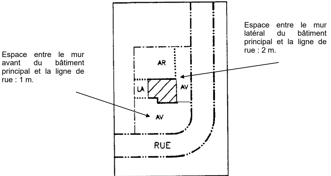
Schéma 1 : Hauteur des clôtures et haies dans la cour avant d'un lot d'angle
